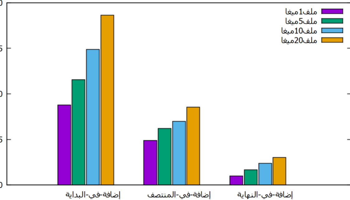
زمن تنفيذ الخوارزمية المقترحة بناءً على مواضع إضافة مختلفة
