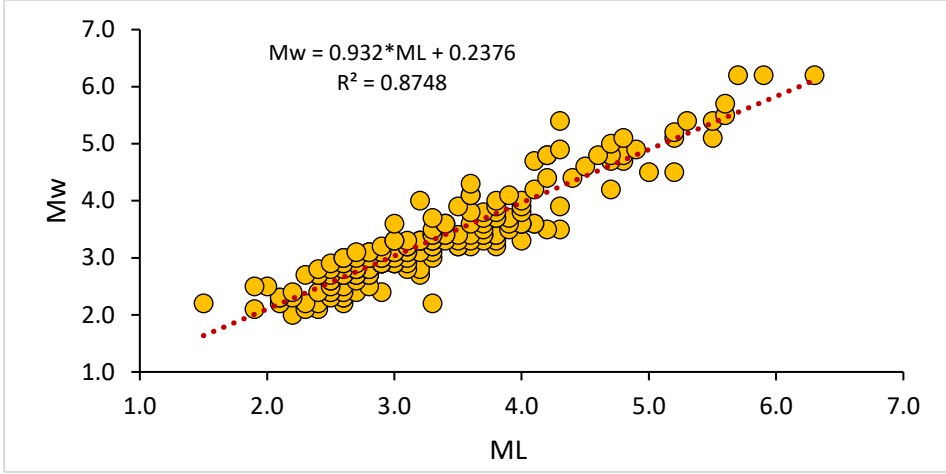
شكل 3. العلاقة التجريبية بين قدر الطاقة ( M_w ) وقدر الهزات المحلية ( M_L ).
