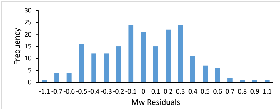
شكل 6. هيستوغرام الفروقات بين قدر الطاقة ( M_w ) المحسوب من العلاقة التجريبية بين قدر الطاقة ( M_w ) والملاحظ في قاعدة معطيات قدر المدة ( M_D ).
