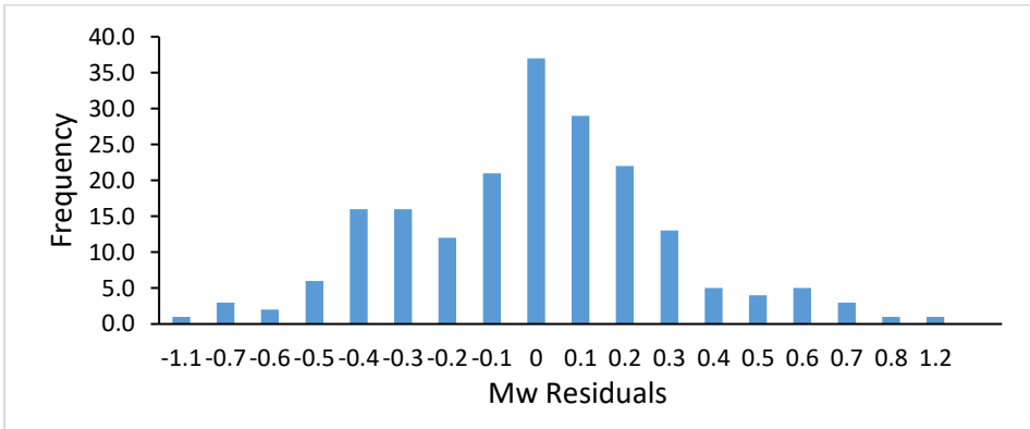
شكل 4. هيستوغرام الفروقات بين قدر الطاقة ( M_w ) المحسوب من العلاقة التجريبية بين قدر الطاقة ( M_w ) والملاحظ في قاعدة المعطيات قدر الهزات المحلية ( M_L ).
