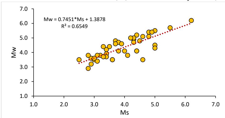
شكل 7. العلاقة التجريبية بين قدر الطاقة ( M_w ) وقدر الأمواج السطحية ( M_s ).
