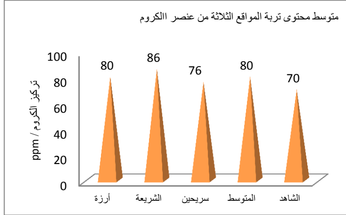
الشكل (2) متوسط محتوى تربة المواقع الثلاثة من عنصر الكروم/ppm
